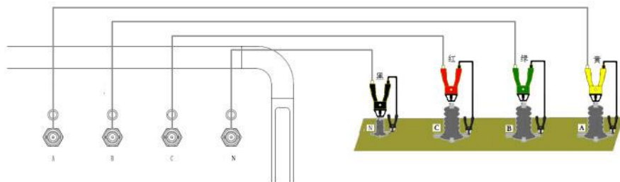
图 2 频响法测试接线图
