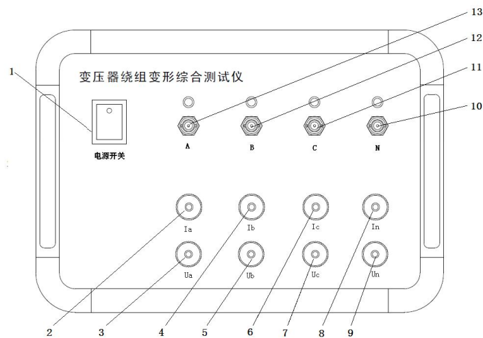
图 1 变压器绕组变形综合测试仪面板图
