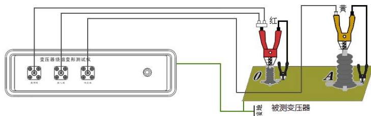
图 2 接线示意图
