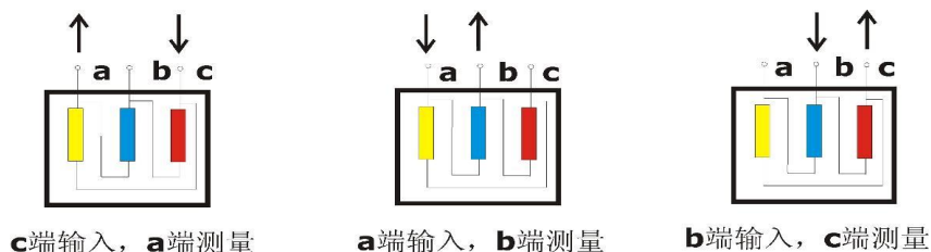
图 5 内连接△接线
