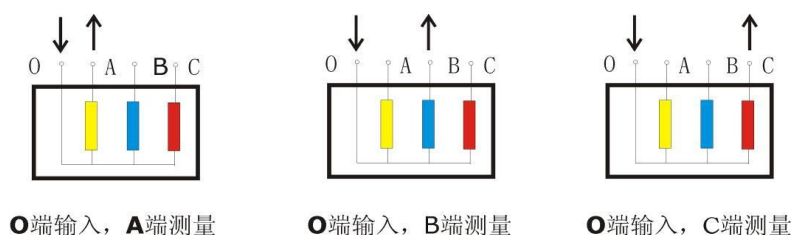
图 3 YN 接线
