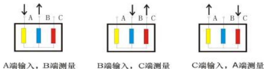
图 4 Y 接线
