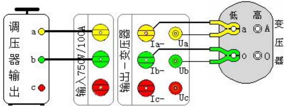
图十四 单相变压器空载试验
