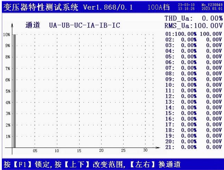
图十三 频谱分析屏
