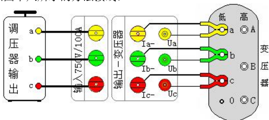
图十八 三相空载测试接线
