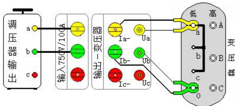
图二十一 零序阻抗测试接线
