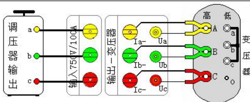
图二十 三相短路测试接线
