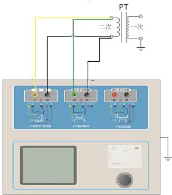
图2.7 PT直阻、励磁试验接线方式
