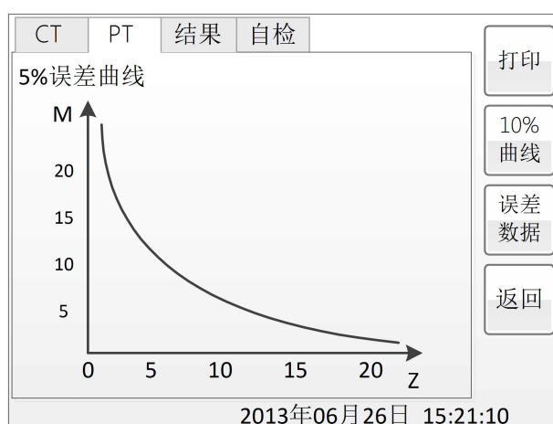
图 2.15 5%误差曲线
