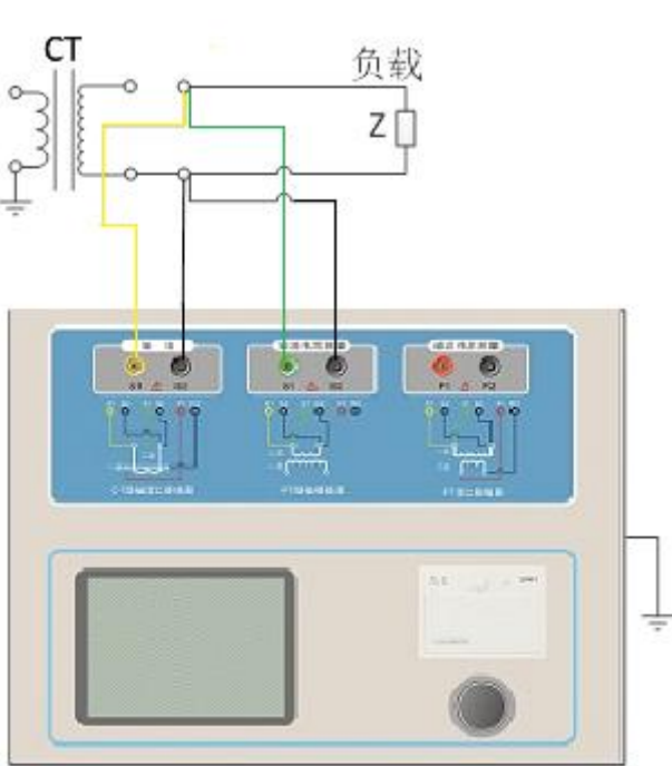
图2.2 CT二次负荷试验接线方式
