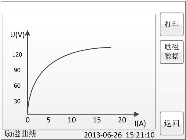
图 2.13 励磁曲线界面
