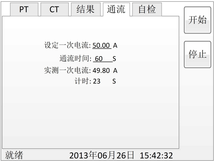
图 2.9 通流试验界面
