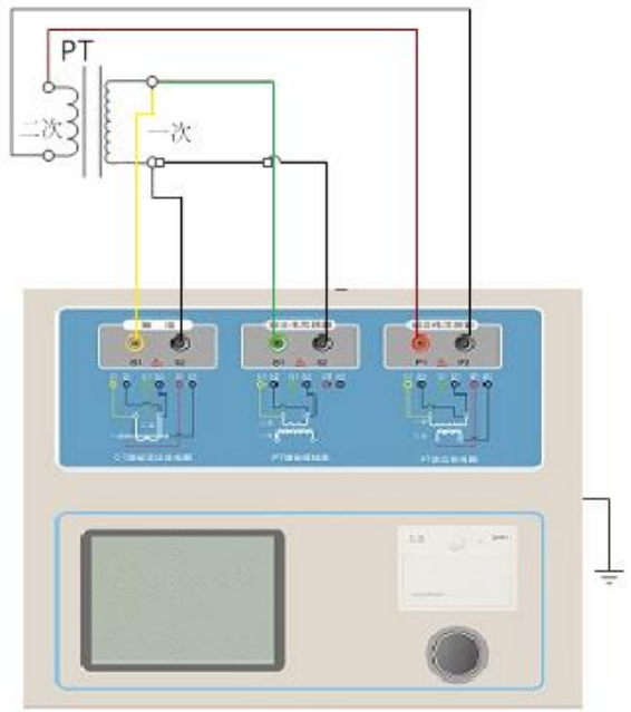
图2.8 PT变比、极性试验接线方式
