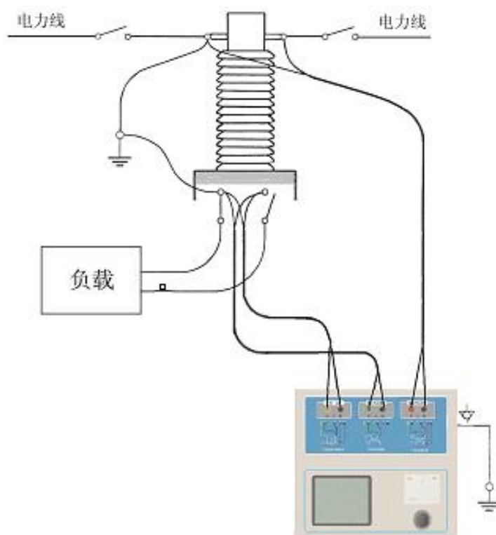
图 C.1 典型接线方式
