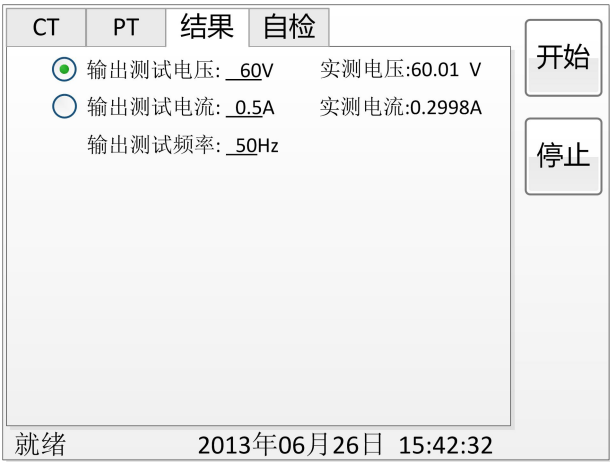
图 2.8 自检测试界面
